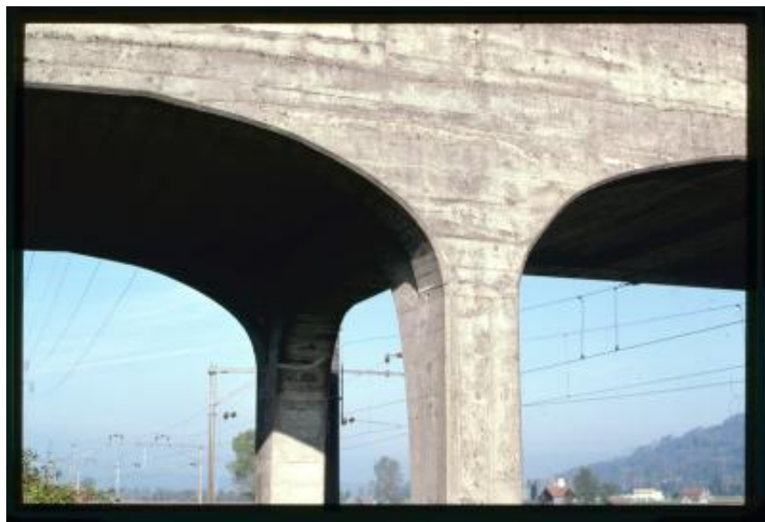
Bilten. Dettaglio delle arcate e dell'intradosso del viadotto attribuibile a Robert Maillart
