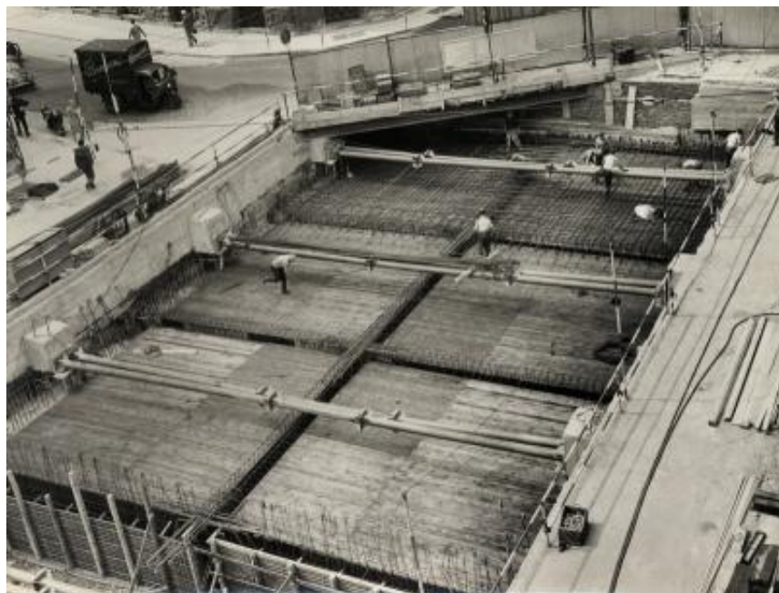
Posa della armatura metallica per la copertura della stazione Palestro a Milano
