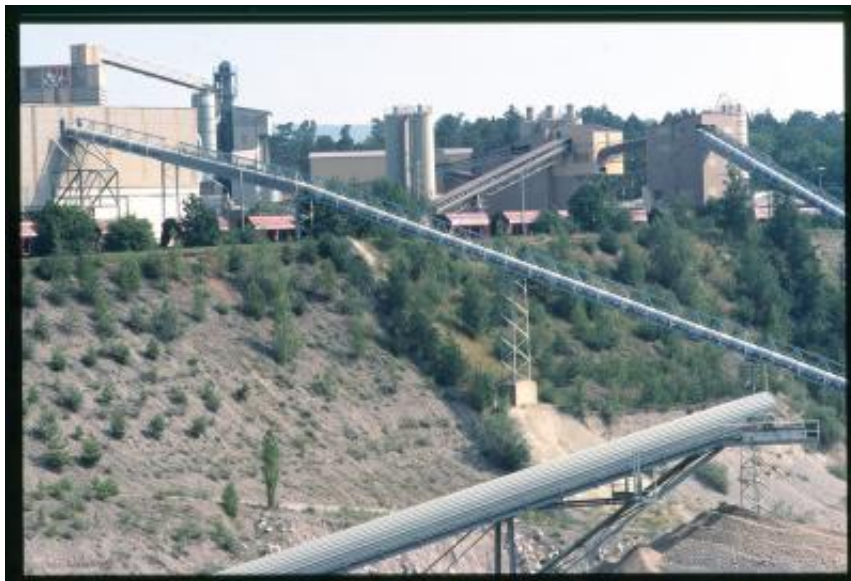
Weiach. Dettaglio delle strutture per l'estrazione della ghiaia di una cava
