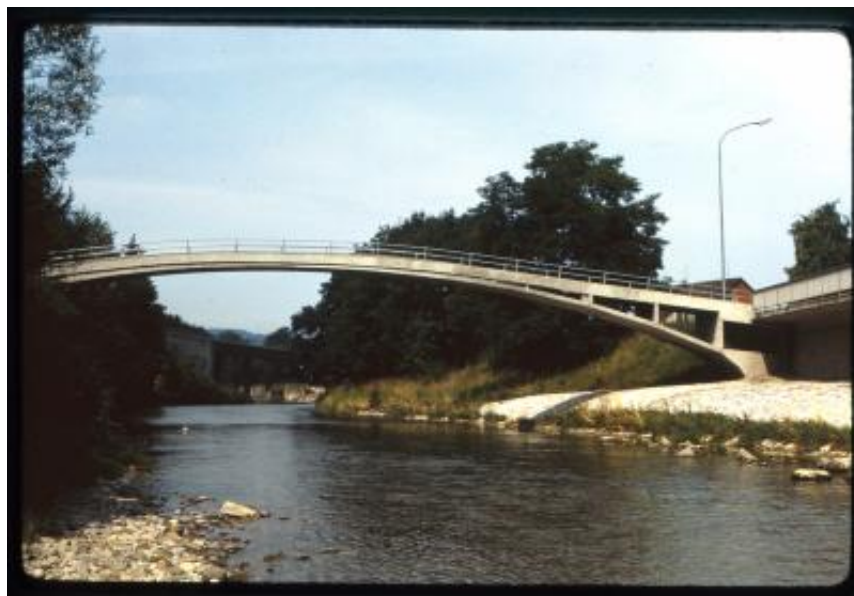
Winterthur. Veduta della passerella sul fiume Töss di Robert Maillart nel distretto di Wülflingen
