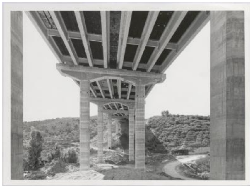
Impalcato prefabbricato utilizzato nella realizzazione dell'autostrada Catania-Messina
