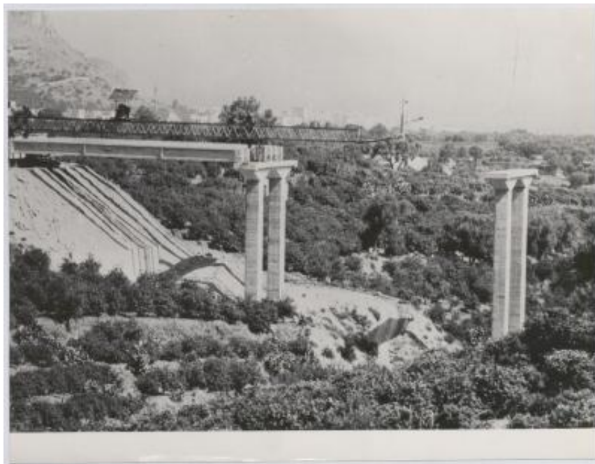
Impalcati prefabbricati utilizzati nella realizzazione dell'autostrada Catania-Messina
