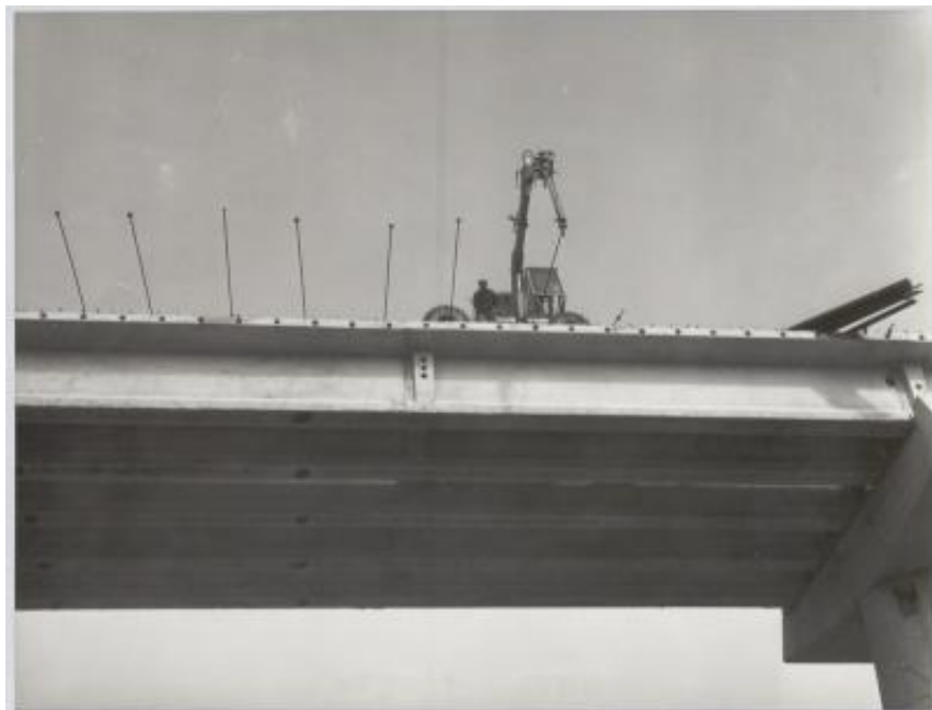
Impalcati prefabbricati utilizzati nella realizzazione dell'autostrada Catania-Messina
