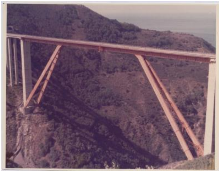
Viadotto sul torrente Sfalassà per l'autostrada Salerno-Reggio Calabria
