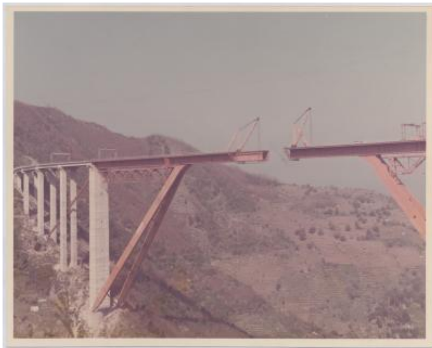
Viadotto sul torrente Sfalassà per l'autostrada Salerno-Reggio Calabria
