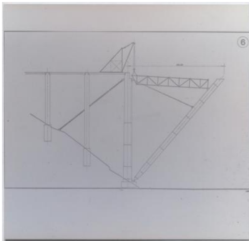
Viadotto sul torrente Sfalassà per l'autostrada Salerno-Reggio Calabria
