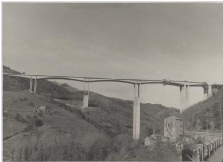
Viadotto sul torrente Gorsexio per l'Autostrada dei Trafori
