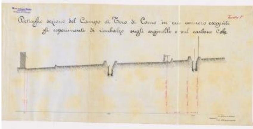
Tavola 1. Dettaglio sezione del Campo di Como in cui vennero eseguiti gli esperimenti di rimbalzo sugli arginelli e sul carbone Coke
