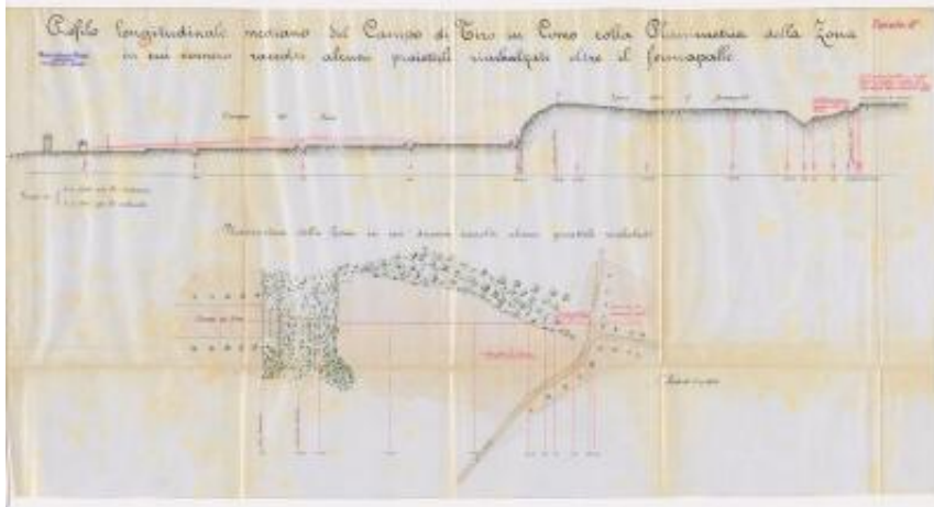
Tavola 2. Profilo longitudinale mediano del Campo di tiro in Como colla planimetria della Zona in cui vennero raccolti alcuni proiettili rimbalzati oltre il fermapalle
