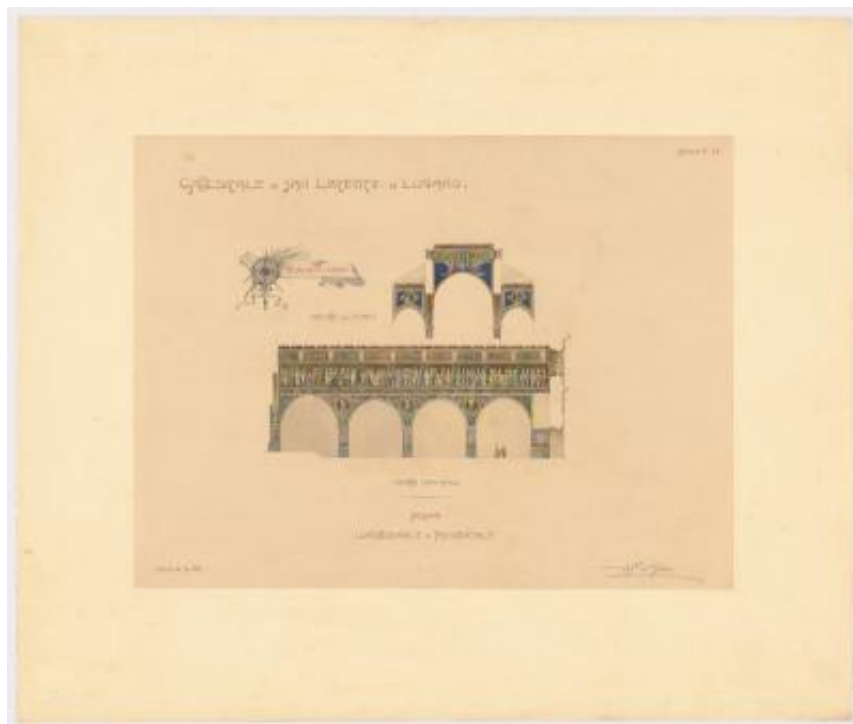
Tavola n. 12. Restauro dell'interno: arcata del coro. Navata principale, sezioni longitudinale e trasversale
