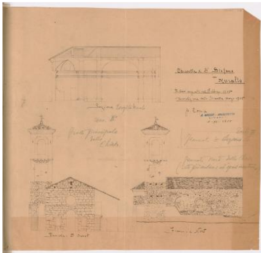
Chiesetta di St. Stefano in Muralto. Rilievi eseguiti nel febbraio 1905
