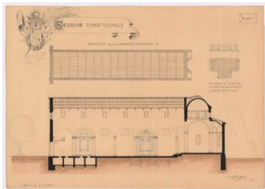
Chiesa di S. Francesco a Locarno. Sezione longitudinale soffitto sulla navata centrale. Tavola 6.
